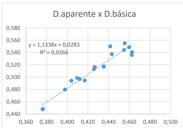
Figura 2. Gráfico de dispersão comparando as densidades aparente e básica da Khaya grandifoliola , valores em g/cm 3 .
