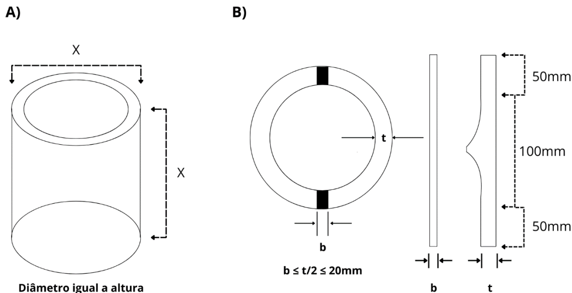
Figura 2. Detalhe das dimensões dos corpos de prova para os ensaios de compressão em “A” e de tração em “B”.
